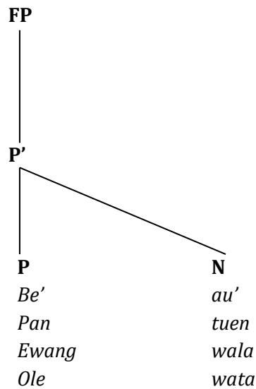
Diagram pohon: 5
