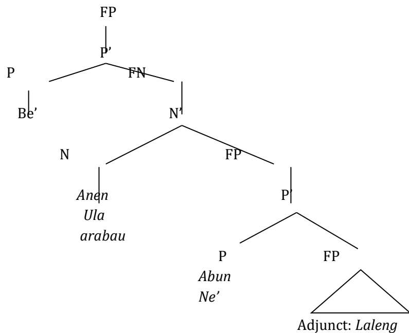
Diagram pohon: 7
